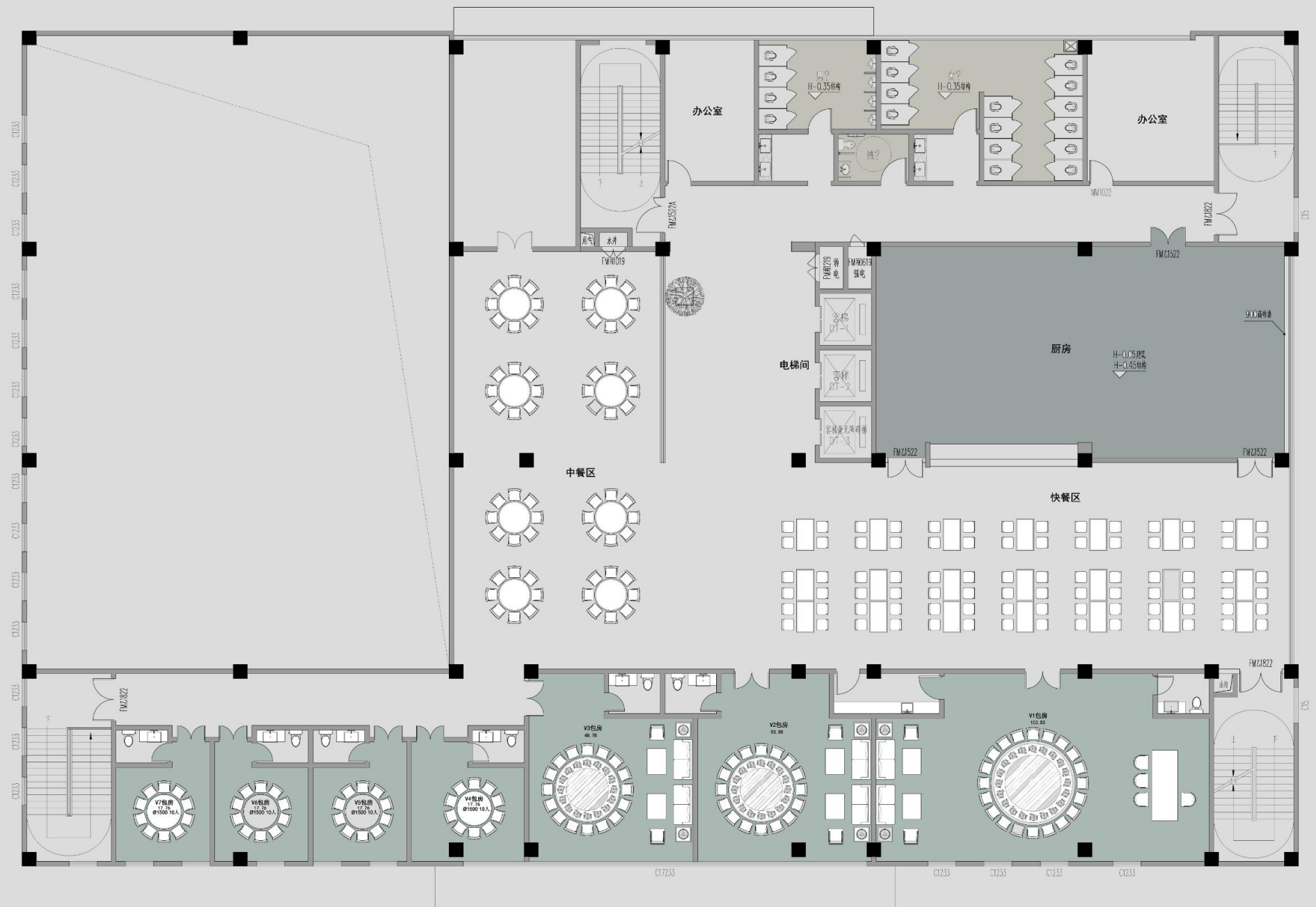
二层平面图
